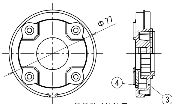
③④継手接続具
